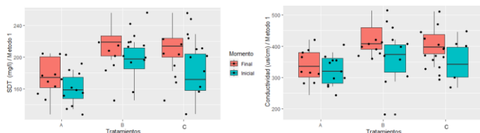
Figura 4. Promedios de SDT y Conductividad de los tratamientos A (humedal con plantas y el contaminante a una concentración específica), B (testigo de las plantas) y C (testigo del contaminante a una concentración puntual) en el método 1; teniendo en cuenta los momentos iniciales y finales
