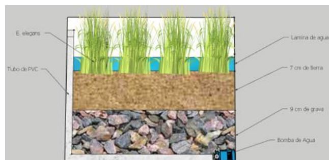
Figura 2. Diseño del humedal artificial con sus respectivos componentes los cuales son grava, tierra, bomba de agua pequeña, tubo de PVC, plantas (en los humedales A y B), agua coloreada (humedal A y C), y agua potable (humedal B).
